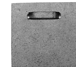
Aufhänge-Bleche , selbstklebend Nr. 25-230 100x100 mm, 8 kg Nr. 25-231 100x200 mm, 12 kg
